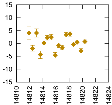
Herstmonceux 7840 AJI CoM (CoM 982 mm) RB 5.5 mm +
