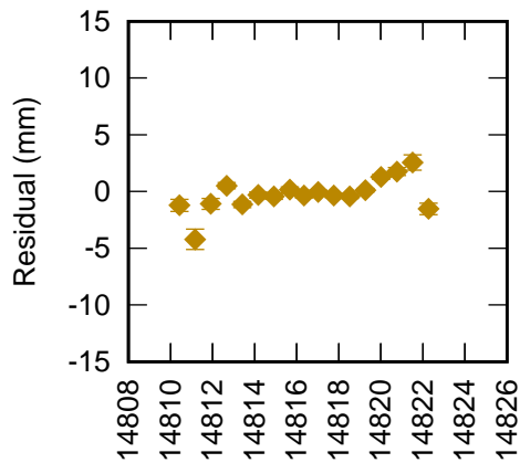
Herstmonceux 7840 LAG1+LAG2 (CoM 245 mm) RB -0.8 mm +
