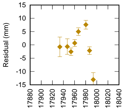
Komsomolsk 1868 LAG1+LAG2 (CoM 248 mm) RB 3.7 mm +
