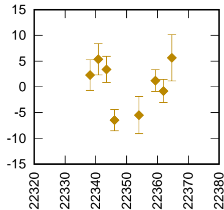
Irkutsk 1891 LARS CoM (CoM 133 mm) RB 9.2 mm +
