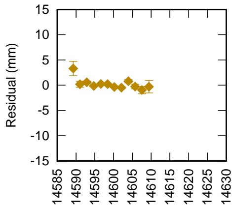
Greenbelt 7105 LAG1+LAG2 (CoM 249 mm) RB -5.2 mm +
