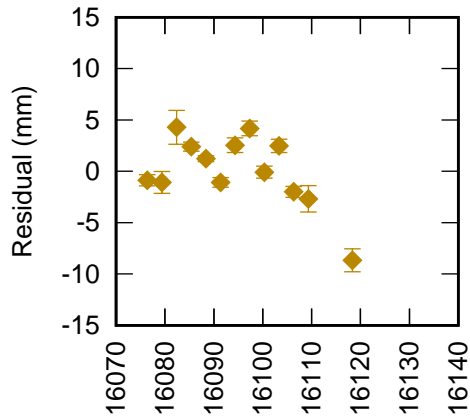
Hartebeesthoek 7501 LAG1+LAG2 (CoM 247 mm) RB 5.1 mm +
