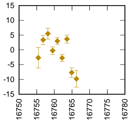
Simosato 7838 STRL+STEL (CoM 75 mm) RB -11.9 mm +
