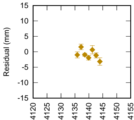
Arequipa 7403 LAG1+LAG2 (CoM 249 mm) RB 18.9 mm +
