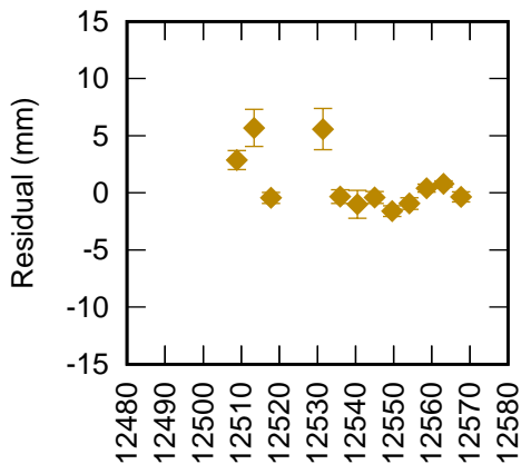
Potsdam 7841 LAG1+LAG2 (CoM 245 mm) RB -0.9 mm +
