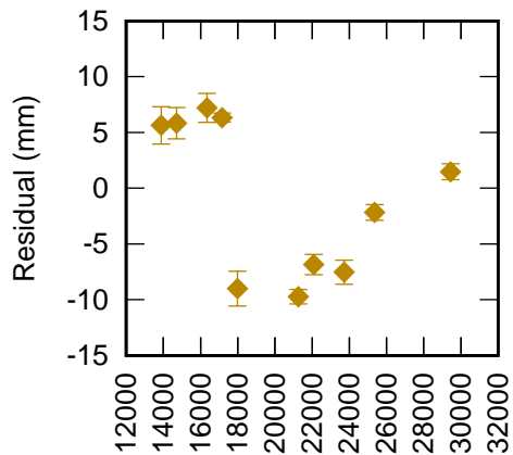
Shanghai 7821 LAG1+LAG2 (CoM 252 mm) RB 1.7 mm +
