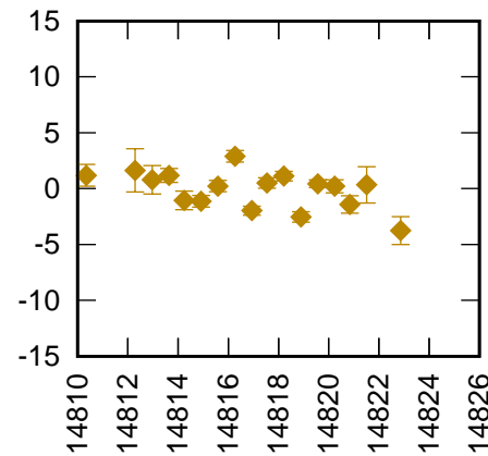
Herstmonceux 7840 LARS CoM (CoM 133 mm) RB 3.8 mm +
