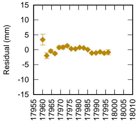
Zimmerwald 7810 LAG1+LAG2 (CoM 249 mm) RB 3.0 mm +
