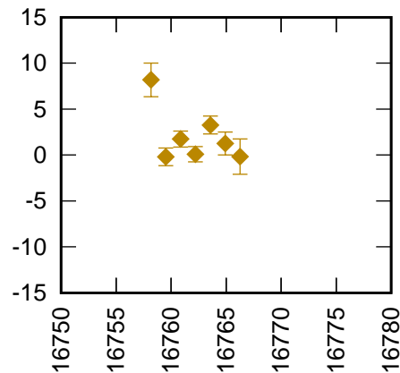
Simosato 7838 LARS CoM (CoM 133 mm) RB -5.9 mm +
