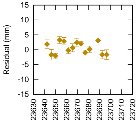
Zelenchukskya 1889 LAG1+LAG2 (CoM 248 mm) RB 17.9 mm +
