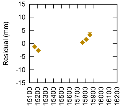
Yarragadee 7090 LAG1+LAG2 (CoM 249 mm) RB 6.2 mm +
