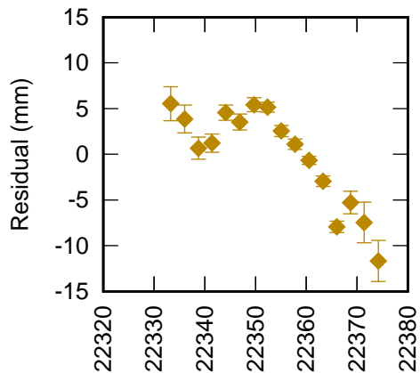
Irkutsk 1891 LAG1+LAG2 (CoM 251 mm) RB 11.3 mm +
