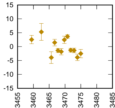
Haleakala 7119 LARS CoM (CoM 133 mm) RB 8.0 mm +
