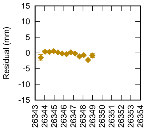
Mt Stromlo 7825 LAG1+LAG2 (CoM 252 mm) RB 10.0 mm +
