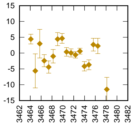
Haleakala 7119 STRL+STEL (CoM 75 mm) RB 8.4 mm +
