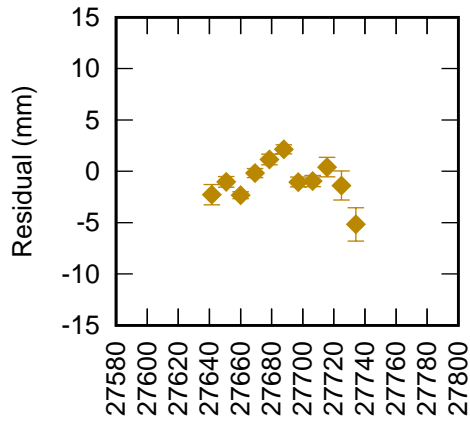
Changchun 7237 LAG1+LAG2 (CoM 252 mm) RB 11.7 mm +
