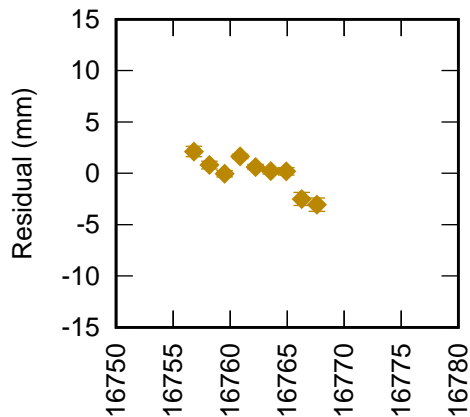
Simosato 7838 LAG1+LAG2 (CoM 250 mm) RB -0.3 mm +
