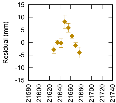
Badary 1890 LAG1+LAG2 (CoM 248 mm) RB 12.1 mm +
