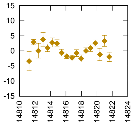
Herstmonceux 7840 STRL+STEL (CoM 75 mm) RB -2.8 mm +
