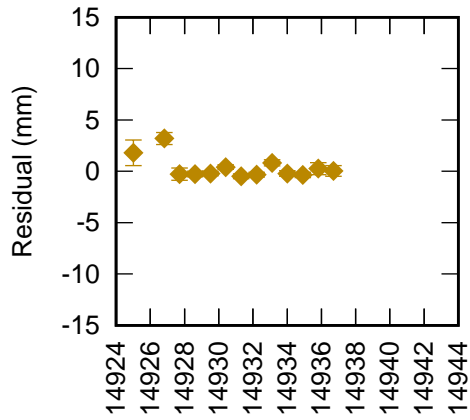
Monument Peak 7110 LAG1+LAG2 (CoM 249 mm) RB 2.3 mm +
