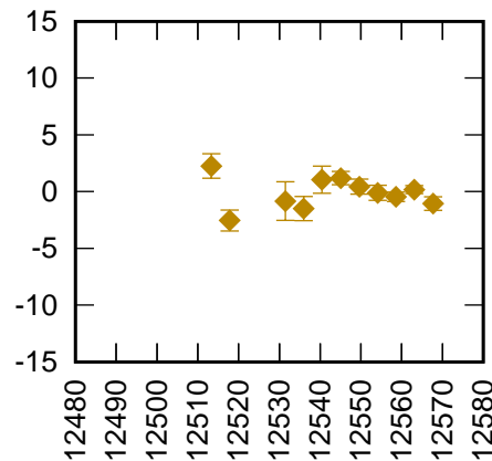
Potsdam 7841 LARS CoM (CoM 133 mm) RB 5.8 mm +
