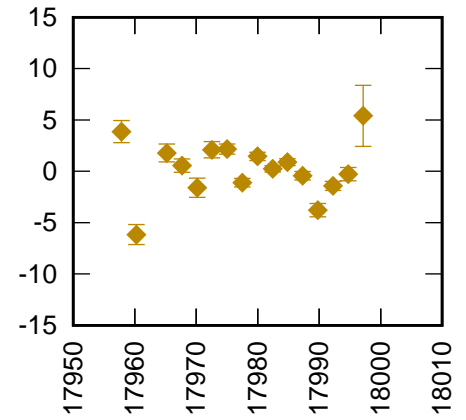
Zimmerwald 7810 LARS CoM (CoM 133 mm) RB 5.1 mm +
