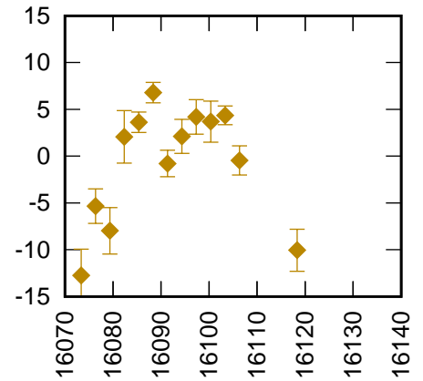
Hartebeesthoek 7501 LARS (CoM 133 mm) RB 10.3 mm +
