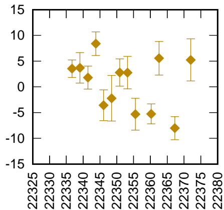
Irkutsk 1891 AJI CoM (CoM 1010 mm) RB 28.8 mm +
