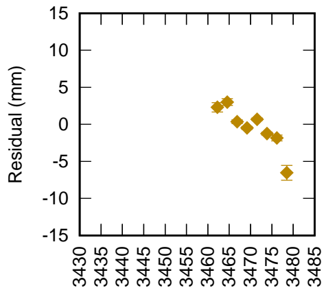
Haleakala 7119 LAG1+LAG2 (CoM 249 mm) RB 14.1 mm +
