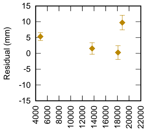
Katzively 1893 LAG1+LAG2 (CoM 246 mm) RB -46.5 mm +
