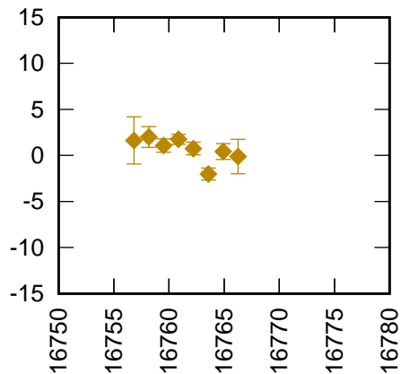
Simosato 7838 AJI CoM (CoM 1016 mm) RB 16.7 mm +
