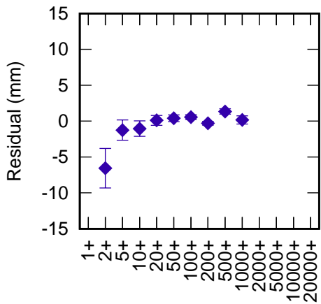
Irkutsk 1891 LAG1+LAG2 (CoM 251 mm) RB 11.3 mm +
