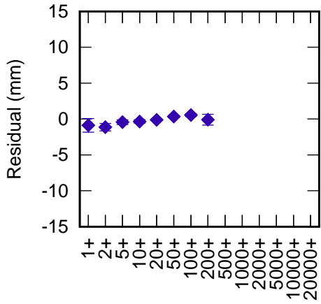
Haleakala 7119 LAG1+LAG2 (CoM 249 mm) RB 14.1 mm +
