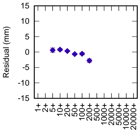
Wetzell 8834 LAG1+LAG2 (CoM 250 mm) RB -19.0 mm +
