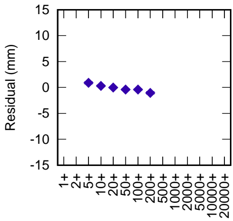
Mt Stromlo 7825 LAG1+LAG2 (CoM 252 mm) RB 10.0 mm +
