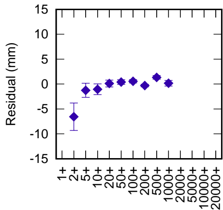
Irkutsk 1891 LAG1+LAG2 (CoM 251 mm) RB 11.3 mm +
