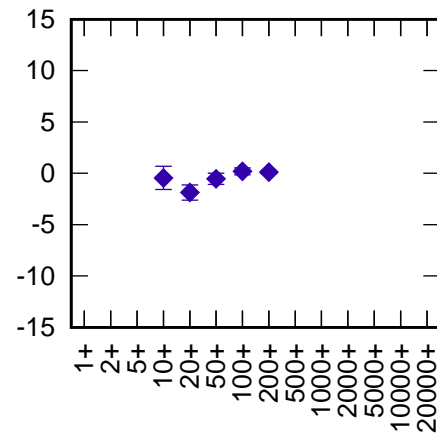
Zimmerwald 7810 LARS (CoM 133 mm) RB 5.1 mm +
