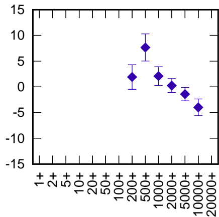
Shanghai 7821 AJI CoM (CoM 1004 mm) RB 2.8 mm +
