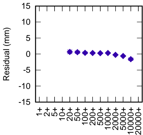
Herstmonceux 7840 LAG1+LAG2 (CoM 245 mm) RB -0.8 mm +
