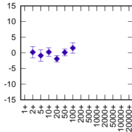
Tahiti 7124 LARS CoM (CoM 133 mm) RB -4.6 mm +
