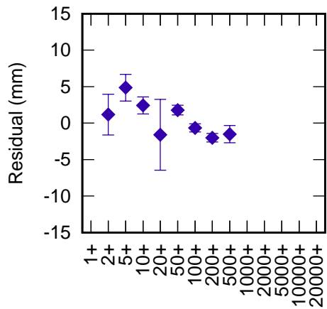
Zelenchukskya 1889 LAG1+LAG2 (CoM 248 mm) RB 17.9 mm +
