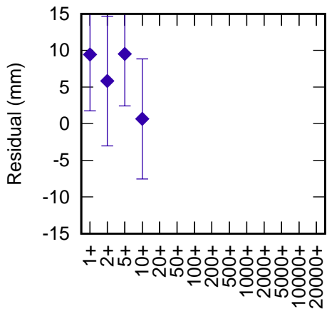
Simeiz 1873 LAG1+LAG2 (CoM 246 mm) RB 3.0 mm +
