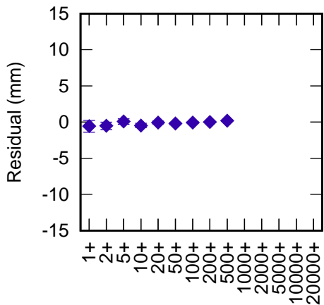
Matera 7941 LAG1+LAG2 (CoM 250 mm) RB -2.5 mm +
