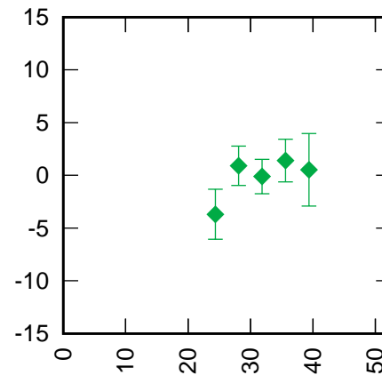
Irkutsk 1891 LARS (CoM 133 mm) RB 9.2 mm +
