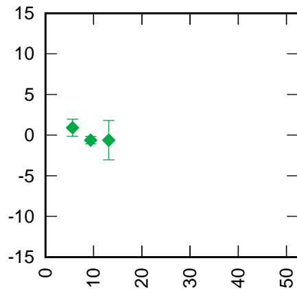
Haleakala 7119 STRL+STEL (CoM 75 mm) RB 8.4 mm +
