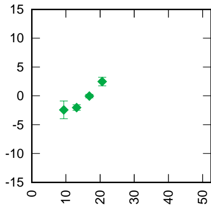
Haleakala 7119 AJI CoM (CoM 1013 mm) RB 39.7 mm +
